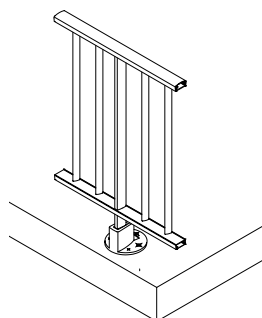
Garde-corps droit à barreaudage Fixation sur dalle
