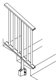
Garde-corps rampant à barreaudage Fixation sur nez de dalle
